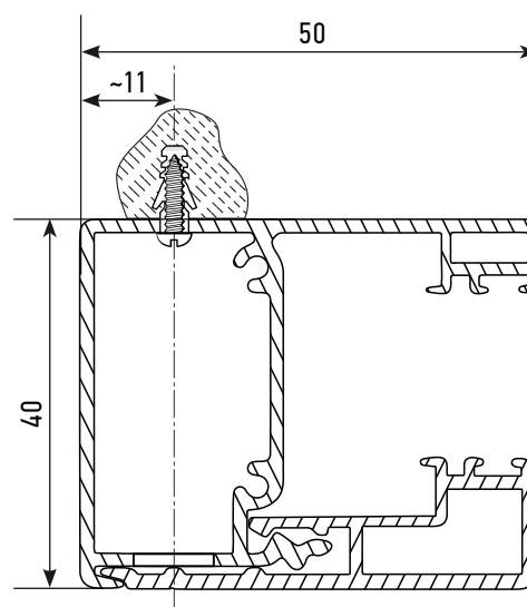
Крепление направляющей ZIP 100 при установке на проем
