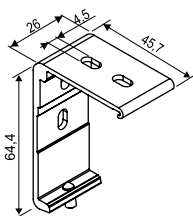
Кронштейн для кассеты М с винтом алюминиевый, белый (опция кронштейн стеновой с винтом)
