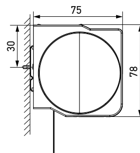
Вид сбоку
