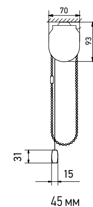
Вид сбоку
