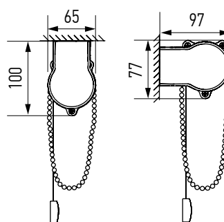
Вид сбоку
