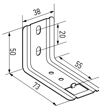
310933-0000 Кронштейн стеновой для кассеты AMG L, 70мм, металл
