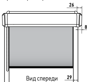
установка короба на шурупы
