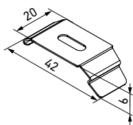
Кронштейн потолочный универсальный М, металл
