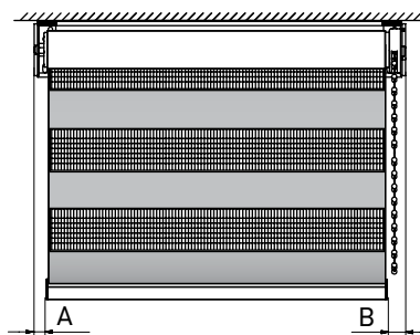
Вид спереди (крепление: потолок)
