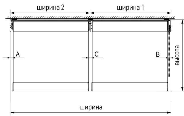
Вид спереди
