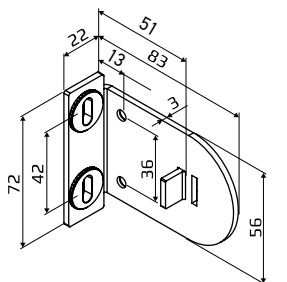
Кронштейн DOUBLE 51 мм L, металл
