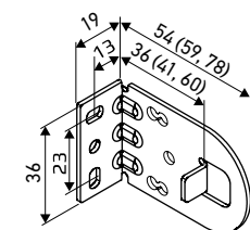
Кронштейн 36 (41, 60) мм M, металл
