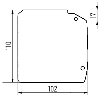
Кассета AMG L Вид сбоку
