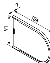
Крышка кронштейна плоская 91x51 мм L для монтажного профиля
